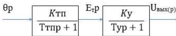
Рисунок 3 - Структурная схема последовательного соединения звеньев
