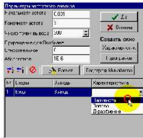
Рисунок 11 - Задание входной и выходной переменных, определяющих фрагмент схемы, для которого будет построен годограф и выбор типа годографа – годограф Найквиста
