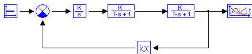
Рисунок 11 - Структурная схема моделирования с И-регулятором
