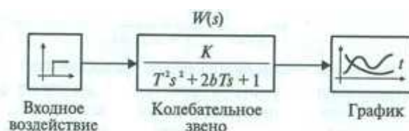
Рисунок 2 - Структурная схема моделирования колебательного звена, изображенная с использованием блоков библиотек ПК «МВТУ»
