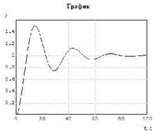
Рисунок 14 - Переходной процесс контура регулирования с И-регулятором K_i=10
