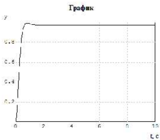
Рисунок 10 - Переходной процесс контура регулирования с П-регулятором K_p=800
