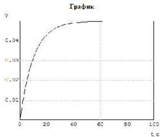
Рисунок 5 - Переходной процесс с начальными условиями (время интегрирования 100)
