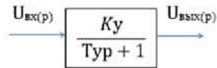
Рисунок 2 - Структурная схема звена с раскрытием передаточной функции и отображением входной и выходной величин
