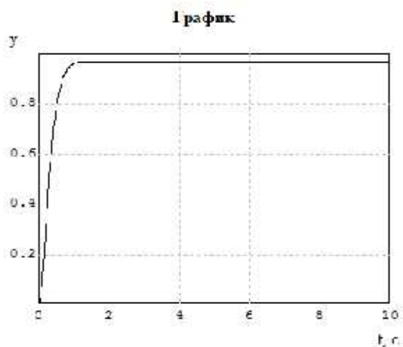
Рисунок 9 - Переходной процесс контура регулирования с П-регулятором K_p=600
