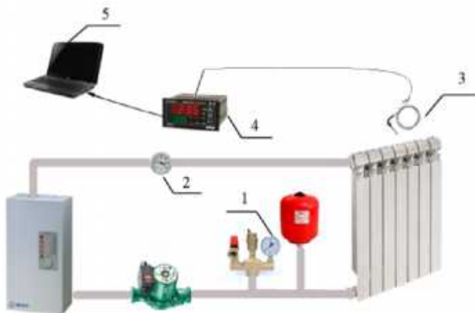
1 - манометр; 2 – термометр; 3 – датчик температуры окружающей среды; 4 – измеритель-регулятор ОВЕН ТРМ 210; 5-ПК с программным обеспечением Owen Process Manager Рисунок 2 – Системы контроля и регулирования системы отопления
