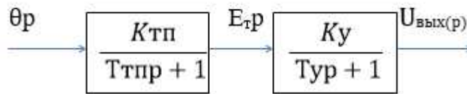
Рисунок 3 - Структурная схема последовательного соединения звеньев
