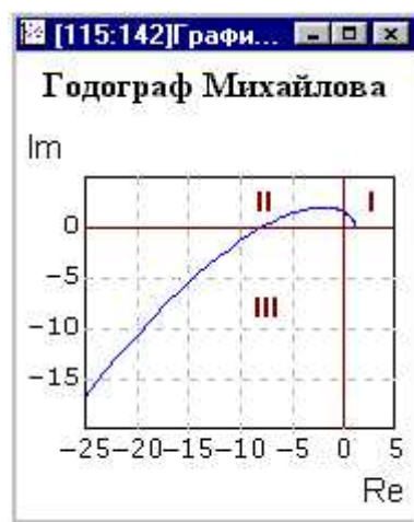
Рисунок 9 - Годограф характеристического полинома разомкнутой САР третьего порядка проходит три квадранта в положительном направлении. Разомкнутая САР устойчива
