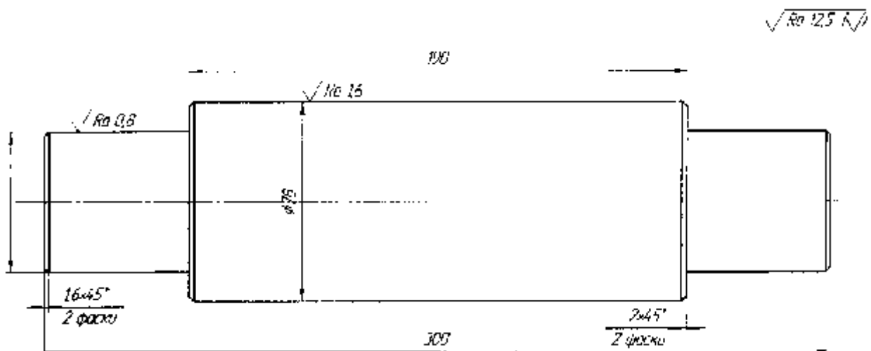
Рисунок 1— Деталь-вал.
