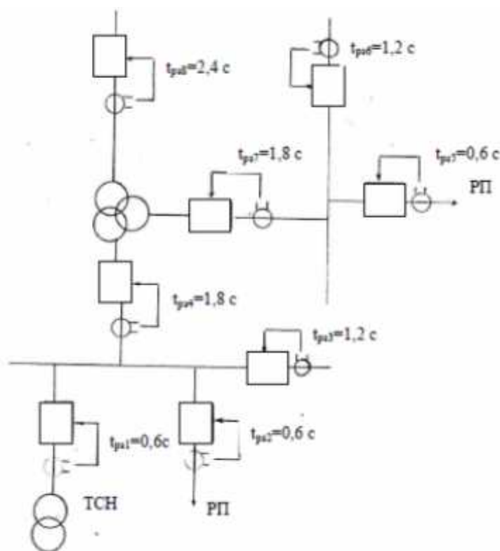
Рисунок 13 - Схема селективности релейных защит
