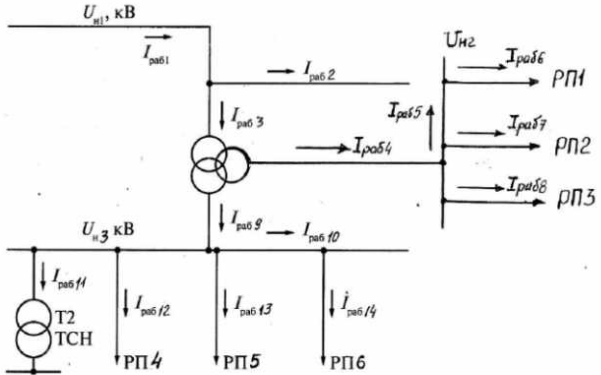
Рисунок 6- Расчетная схема для определения рабочих токов
