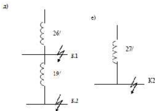
Рисунок 9 – Схемы преобразования
