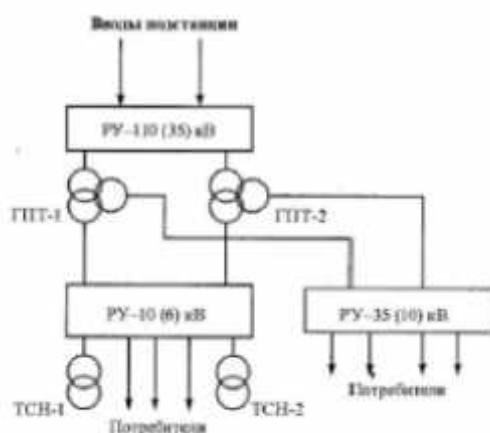
Рисунок 2 – Структурная схема трансформаторной подстанции с тремя уровнями вторичного напряжения
