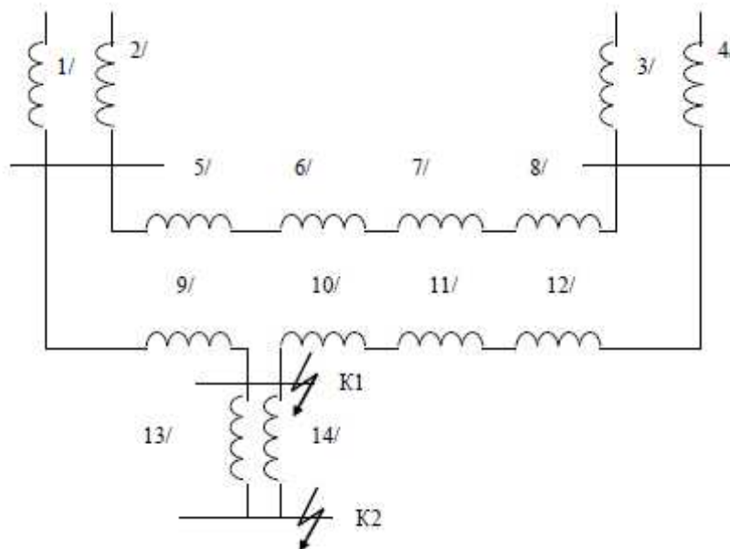
Рисунок 8 - Схема замещения для определения токов короткого замыкания для транзитной подстанции
