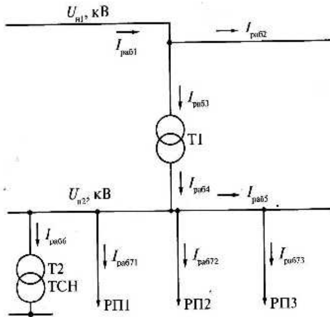
Рисунок 4 - Расчетная схема для определения рабочих токов
