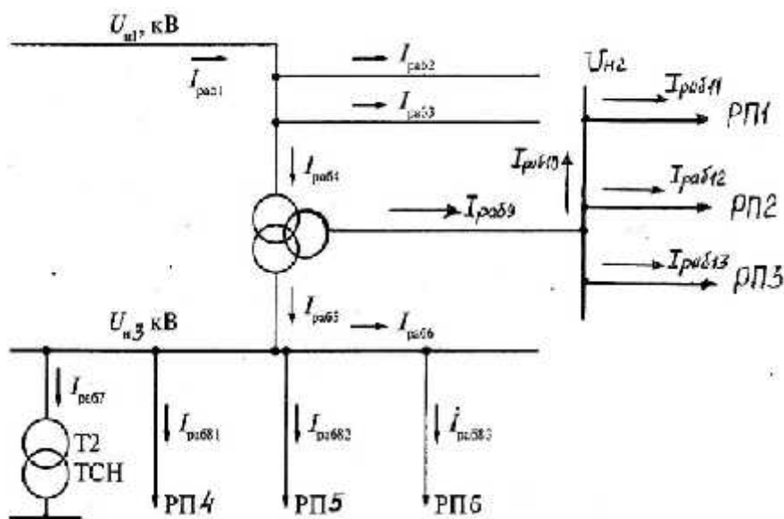
Рисунок 5 - Расчетная схема для определения рабочих токов
