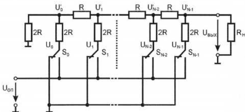
Рис. 11.2. ЦАП с инверсным включением резистивной матрицы
