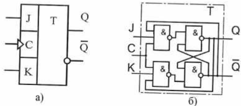
Рис. 5.4. Условное графическое обозначение однотактного JK -триггера (а) и его логическая структура (б)
