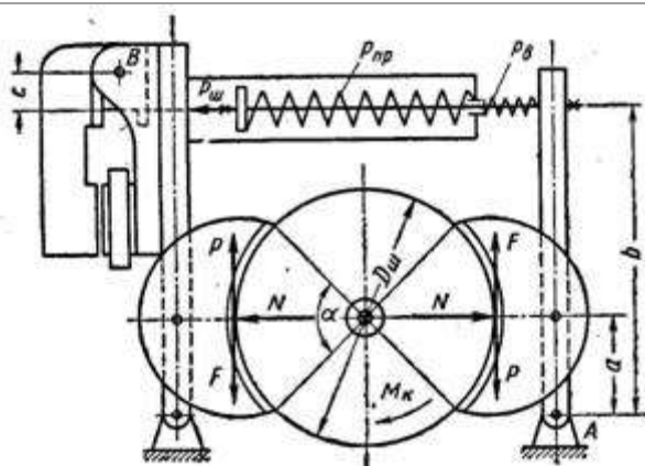
Схема к расчету двухколодочного пружинного тормоза
