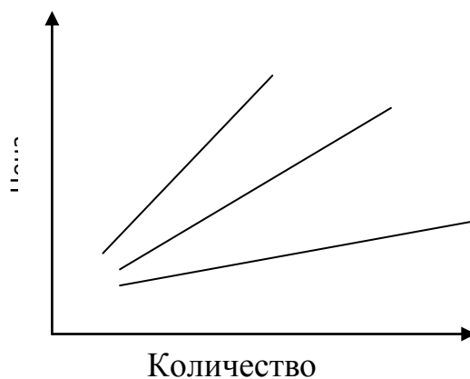
Рисунок 2 - Кривые предложения S^0 , S^1 , S^2
