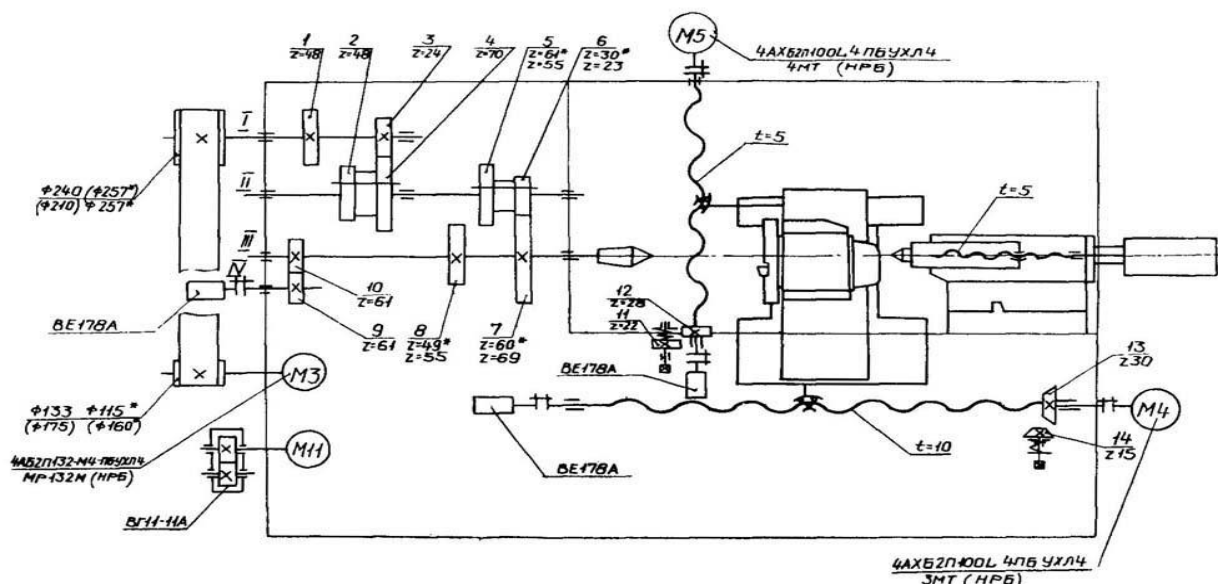
Рис. 21. Кинематическая схема цифры в скобках для привода НПБ.
